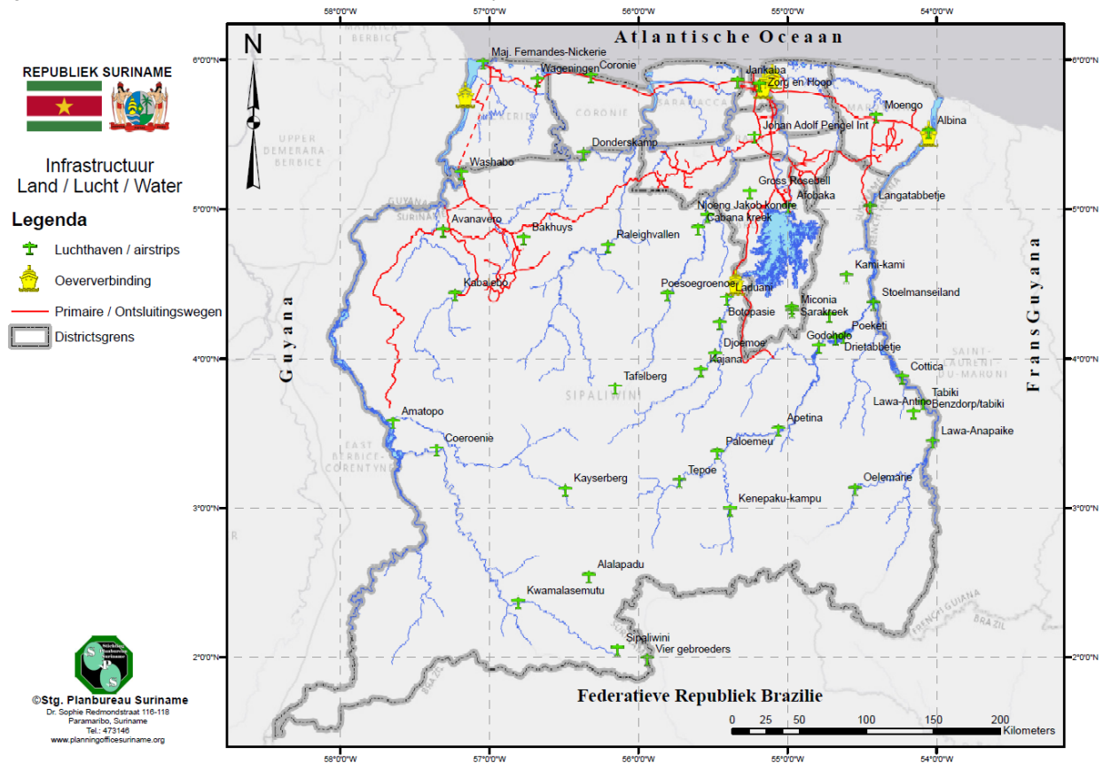
Figuur A6.17.1: Primaire land-, lucht- en waterinfrastructuur
